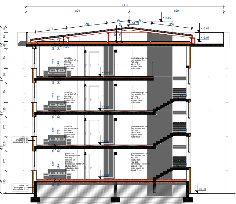
PRESEK 2-2
