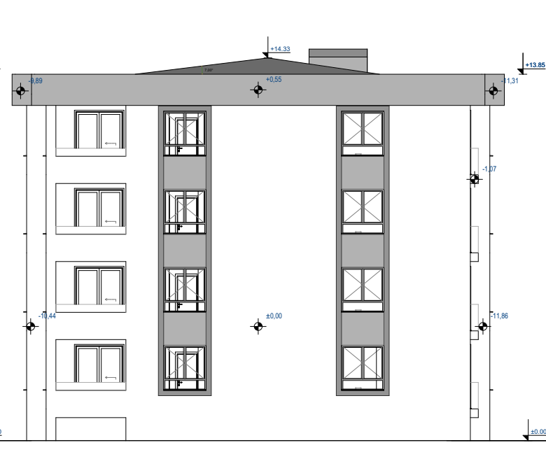
SEVEROZAPADNA FASADA
