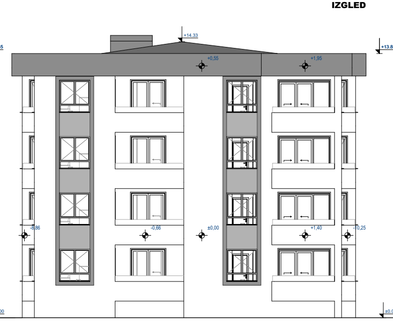
JUGOISTOČNA FASADA
