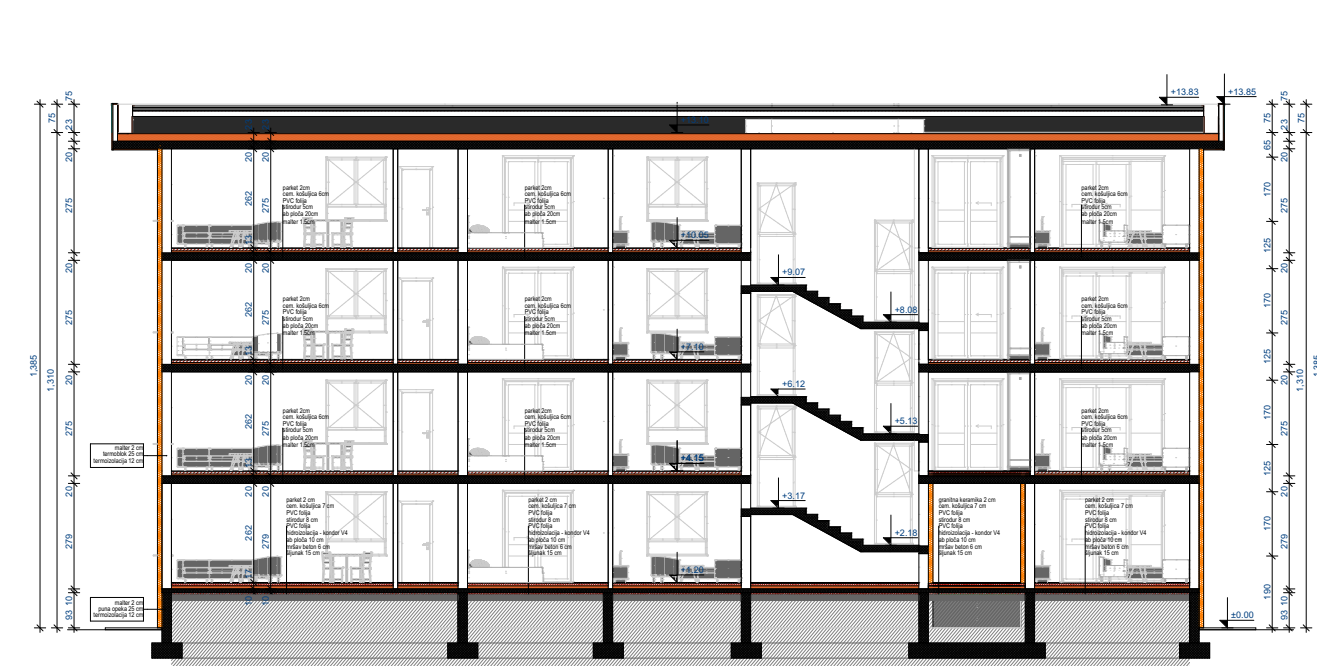
PRESEK 4-4
