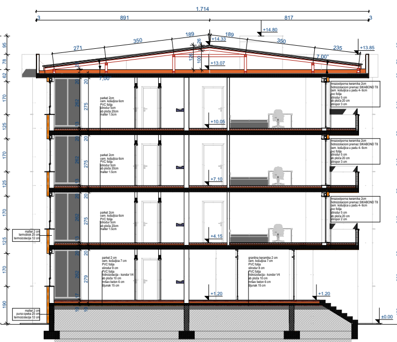
PRESEK 1-1
