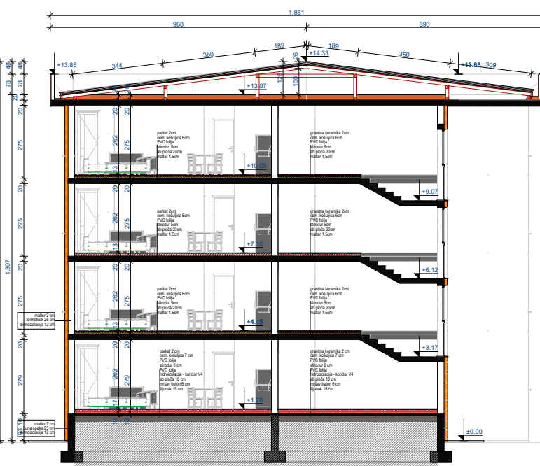
PRESEK 3-3
